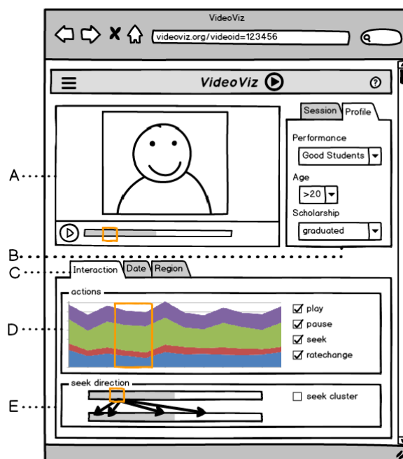
Figura 1: Esboço da ferramenta VideoViz
