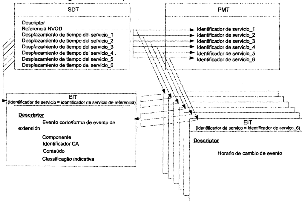
Figura B.3 Descripción de un servicio NVOD en el SI
