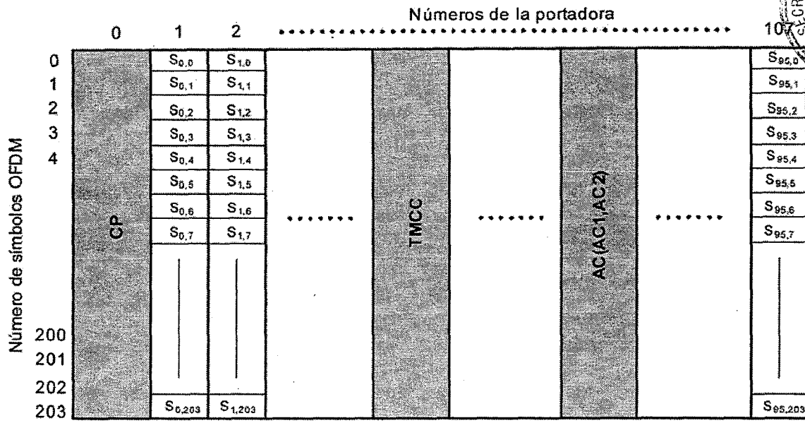
Figura 32. Configuración del segmento OFDM para modulación diferencial
