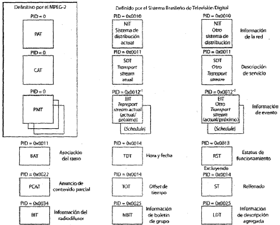
Figura 77. Estructura de las señales de control de la transmisión
