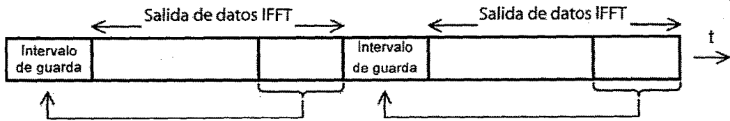
Figura 36. Inserción de intervalo de guarda
