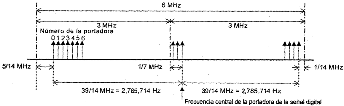
Figura 37. Ejemplo del arreglo de portadoras de la señal OFDM para la señal de televisión digital terrestre
