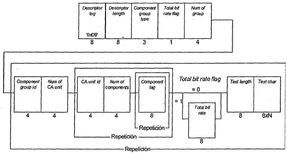
Figura 60. Estructura de datos del descriptor de grupo de componentes
