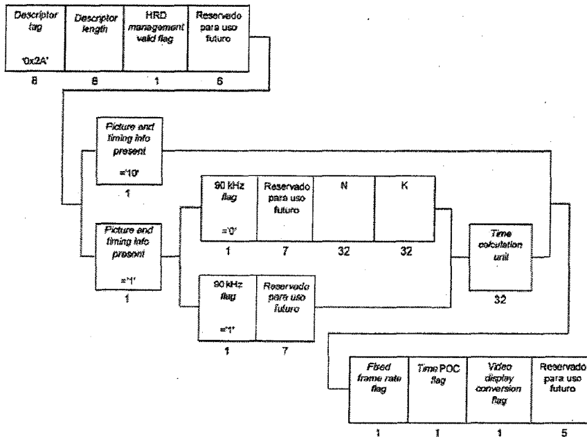
Figura 71. Estructura de datos del descriptor para AVC timing y para el decodificador hipotético de referencia (HRD)
