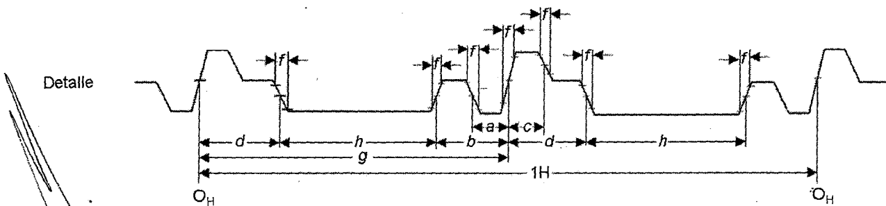
Figura 13. Señales de sincronismo de campo para 1125/59,94/50/2:1
