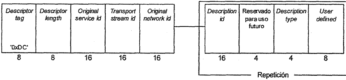
Figura 63. Estructura de datos del descriptor de conexión de la LDT
