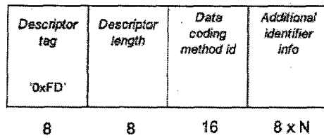
Figura 37. Estructura de datos del descriptor de componente de datos
