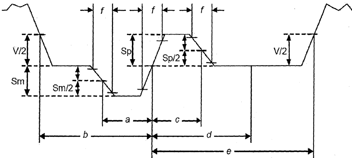
Figura 9. Señal de sincronismo de línea para 1125/59,94/50/2:1
