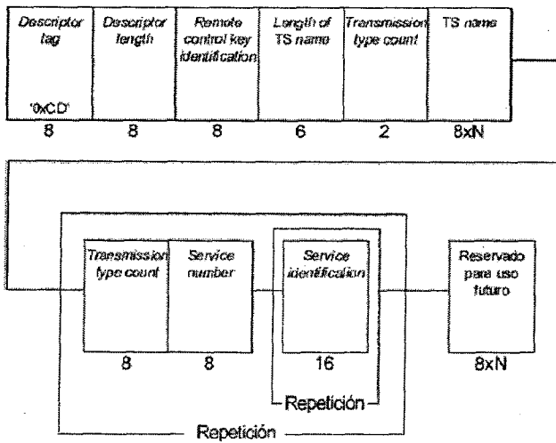
Figura 65. Estructura de datos del descriptor de informaciones del TS
