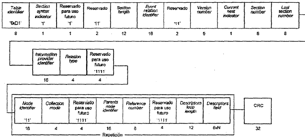
Figura 14. Estructura de datos de la ERT
