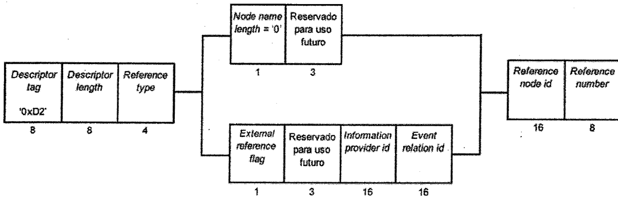
Figura 51. Estructura de datos del descriptor de node relation
