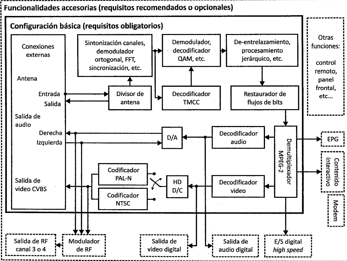
Figura 2-Configuración básica del IRD tipo convertidor digital (STB)
