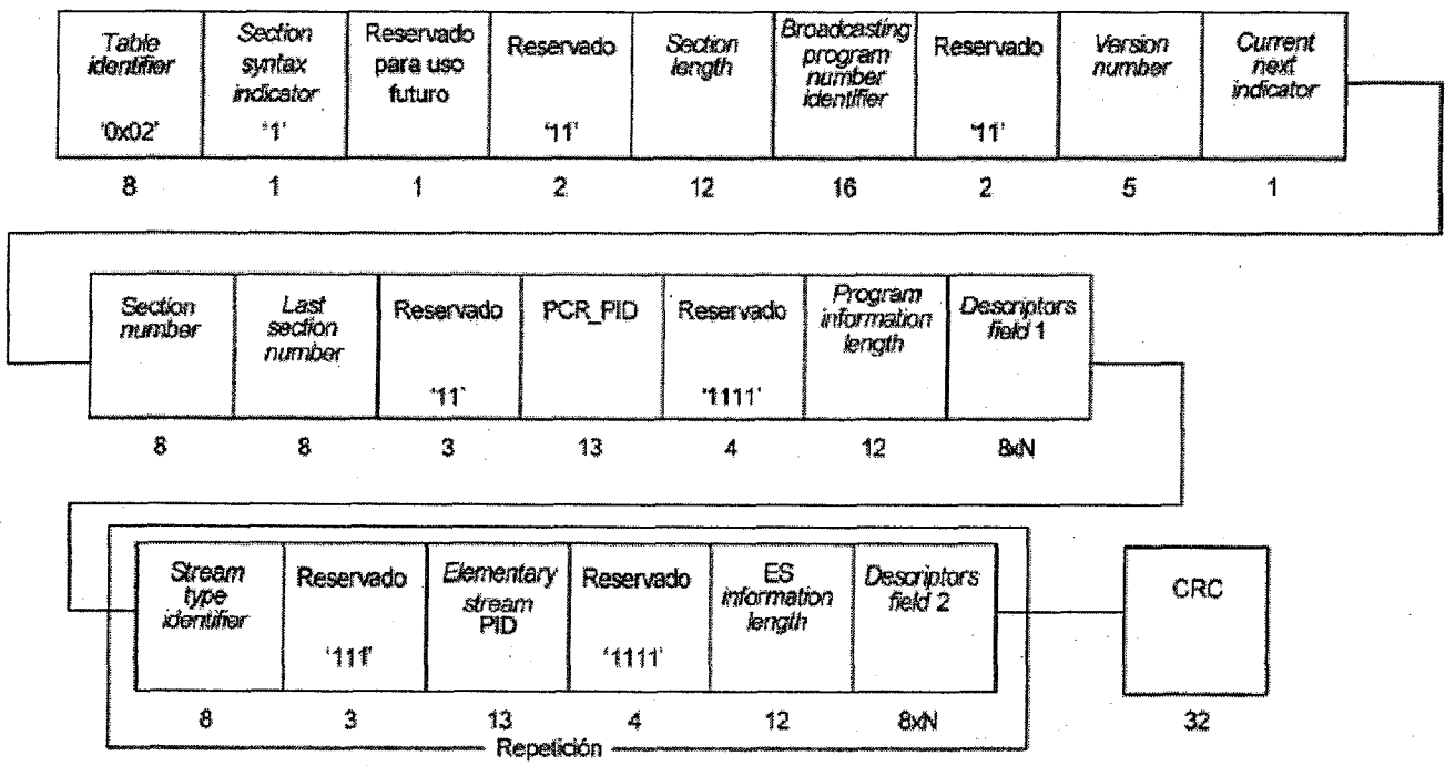
Figura 2. Estructura de datos de la PMT
