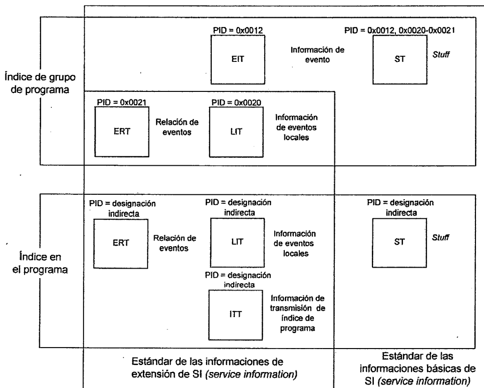
Figura 81. Organización de las informaciones de extensión de la SI
