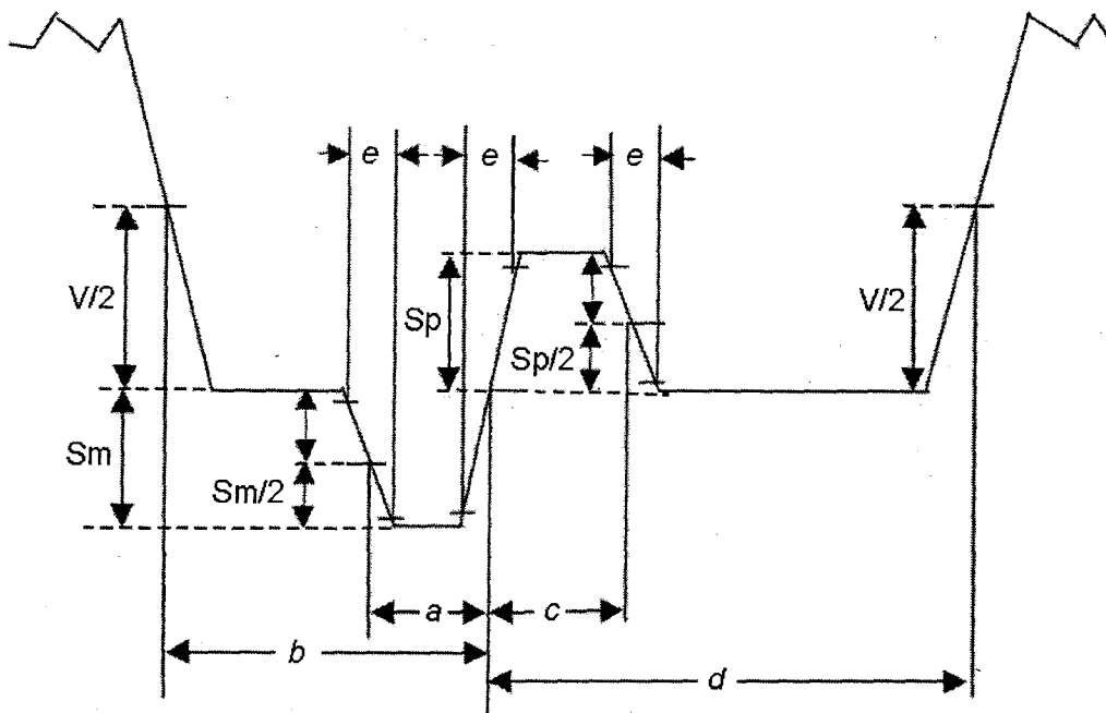
Figura 8. Señal de sincronismo de línea para 750/59,94/50/1:1
