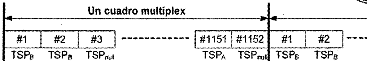
Figura 5. Ejemplo de un TS remultiplexado (modo 1, intervalo de guarda 1/8)
