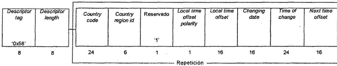
Figura 43. Estructura de datos del descriptor de diferencia de huso
