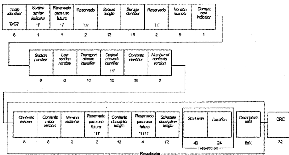
Figura 12. Estructura de datos de la PCAT
