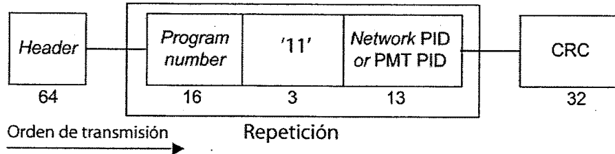
Figura 25. Tabla de asociación de programa
