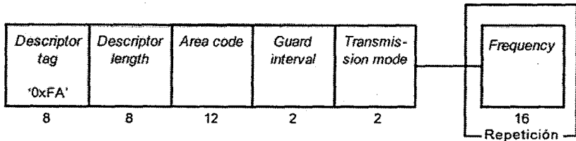
Figura 54. Estructura de datos del descriptor de distribución terrestre
