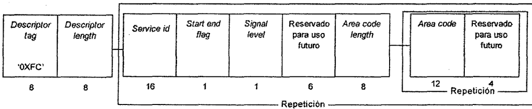
Figura 42. Estructura de datos del descriptor de información de emergencia
