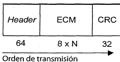
Figura 29. Estructura y procedimiento de transmisión del ECM
