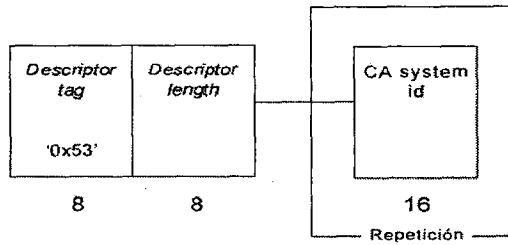
Figura 34. Estructura de datos del descriptor identificador de CA
