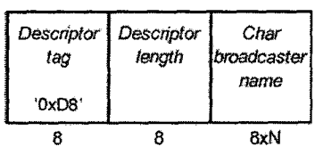
Figura 59. Estructura de datos del descriptor de nombre del radiodifusor
