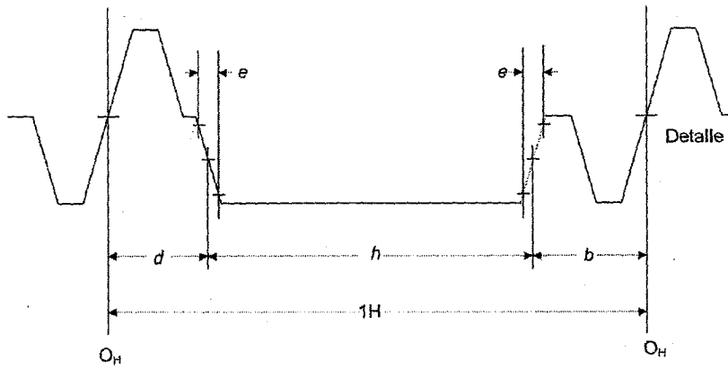
Figura 12. Señales de sincronismo de campo para 750/59,94/50/1:1
