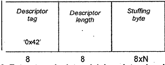
Figura 22. Estructura de datos del descriptor de relleno (stuffing)
