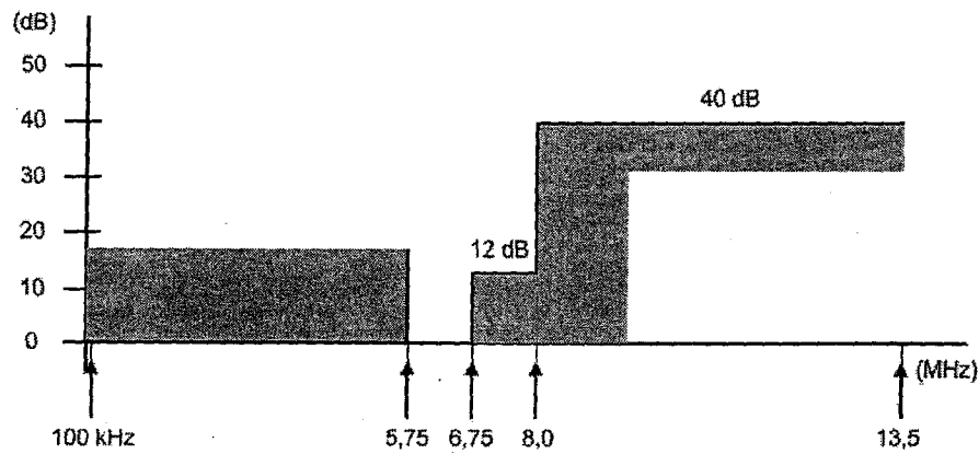
Figura 1. Características de atenuación vs. frecuencia para la señal de luminancia en los filtros del sistema 525/59,94/2:1 y 625/50/2:1(atenuación relativa a la de 100 kHz)
