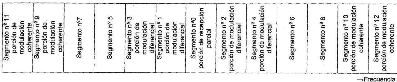
Figura 35. Numeración de los segmentos OFDM en el espectro de transmisión y ejemplo de uso
