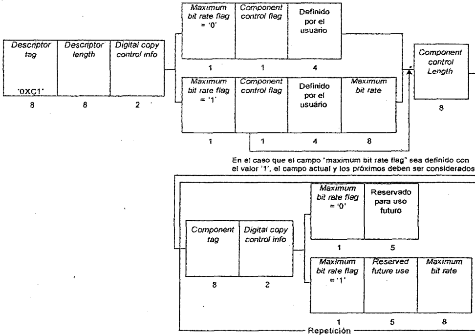
Figura 41. Estructura de datos del descriptor de control de copias digitales
