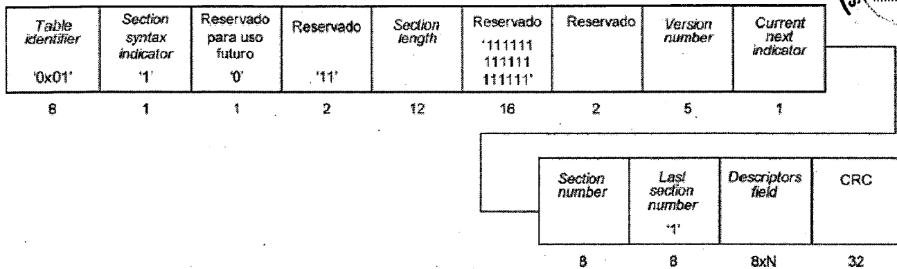
Figura 3. Estructura de datos de la CAT
