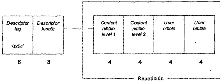
Figura 35. Estructura de datos del descriptor de contenido
