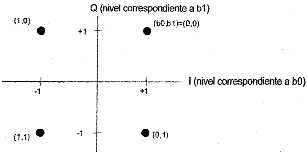
Figura 17. Constelación QPSK
