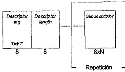
Figura 69. Estructura de datos del descriptor de composición del carrusel de datos
