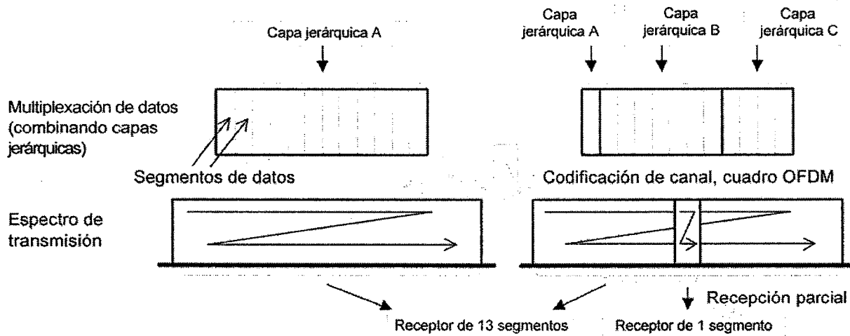
Figura 3. Ejemplo de transmisión jerárquica y recepción parcial
