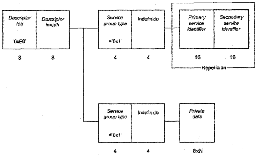
Figura 72. Estructura del descriptor de grupo de servicio
