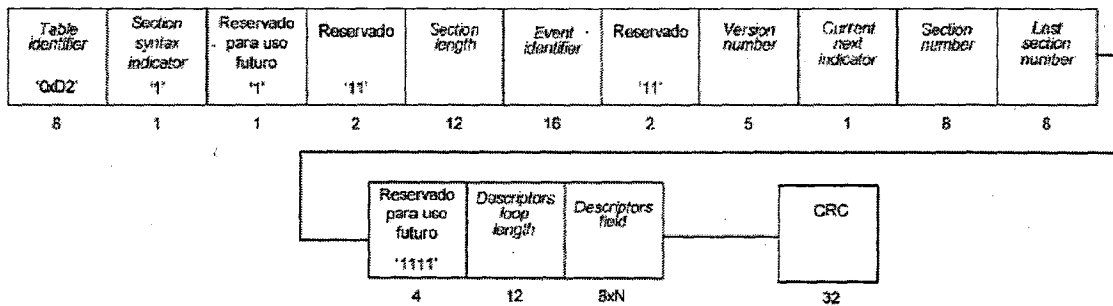
Figura 15. Estructura de datos de la ITT
