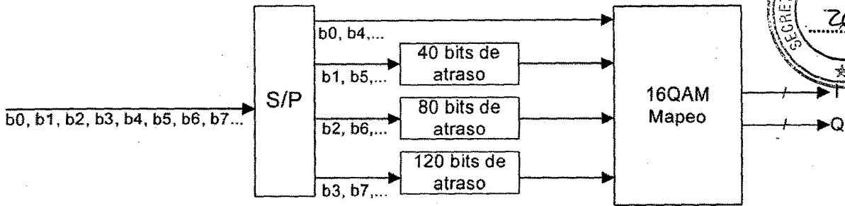
Figura 18. Diagrama del sistema de modulación 16QAM
