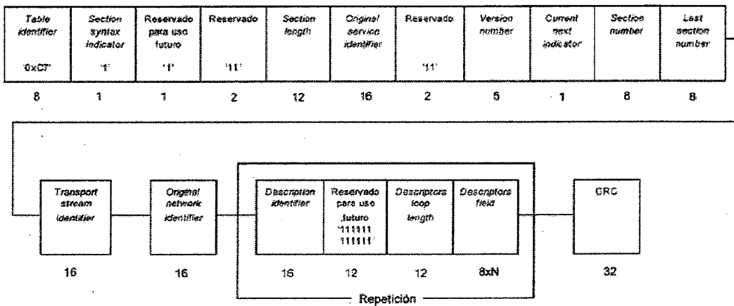
Figura 18. Estructura de datos de la LDT
