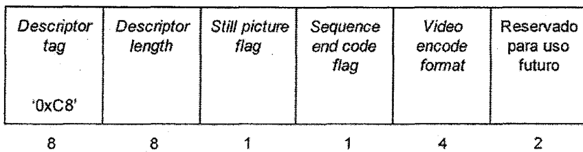
Figura 48. Estructura de datos del descriptor de control de decodificación de video
