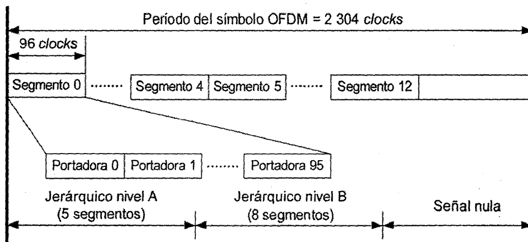
Figura 7. Ejemplo de organización del tiempo para la señal de entrada para la capa jerárquica
