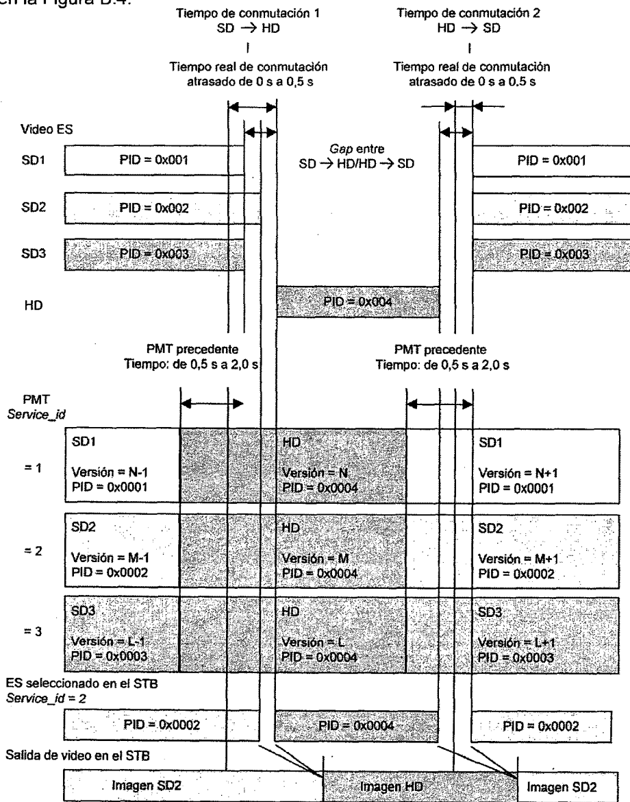
Figura B.4 Carta de mapeo de tiempo de una conmutación seamless
