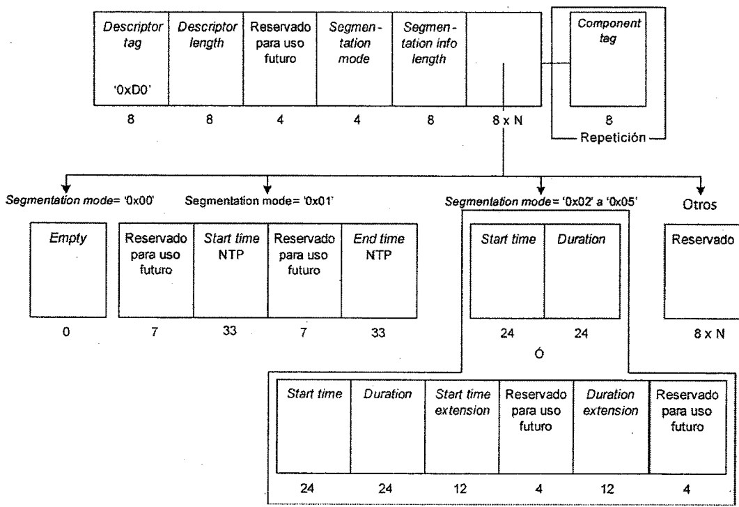
Figura 49. Estructura de datos del descriptor de eventos locales básicos
