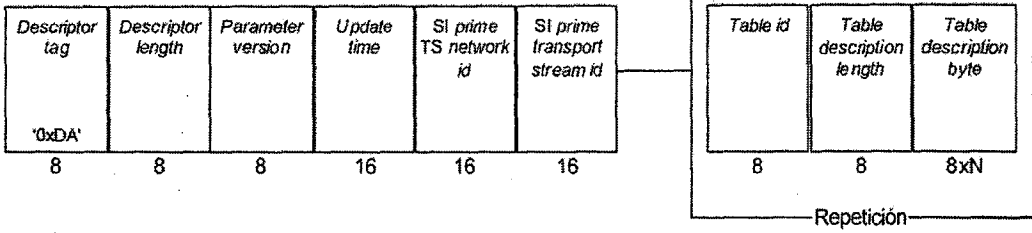
Figura 61. Estructura de datos del descriptor del principal TS del SI
