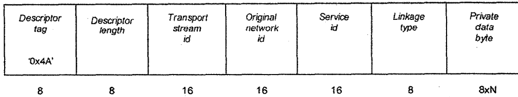
Figura 26. Estructura de datos del descriptor de conexiones
