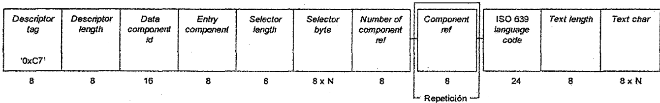
Figura 47. Estructura de datos del descriptor de contenido de datos
