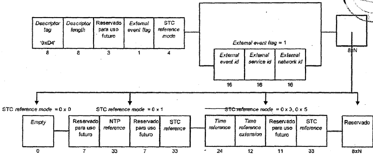
Figura 53. Estructura de datos del descriptor para la referencia de reloj del sistema (system time clock)
