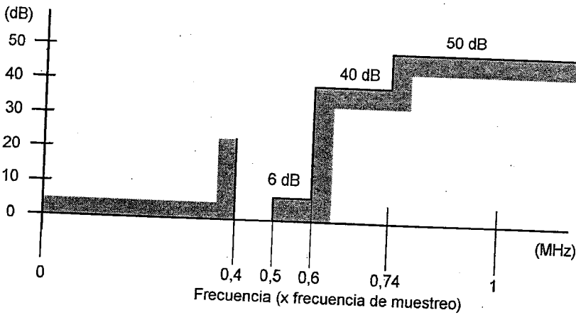
Figura 6. Características de atenuación vs. frecuencia para las señales de complemento de color en los filtros de los sistemas 750/59,94/50/1:1 y 1125/59,94/50/2:1 (atenuación relativa a la de 100 kHz)
