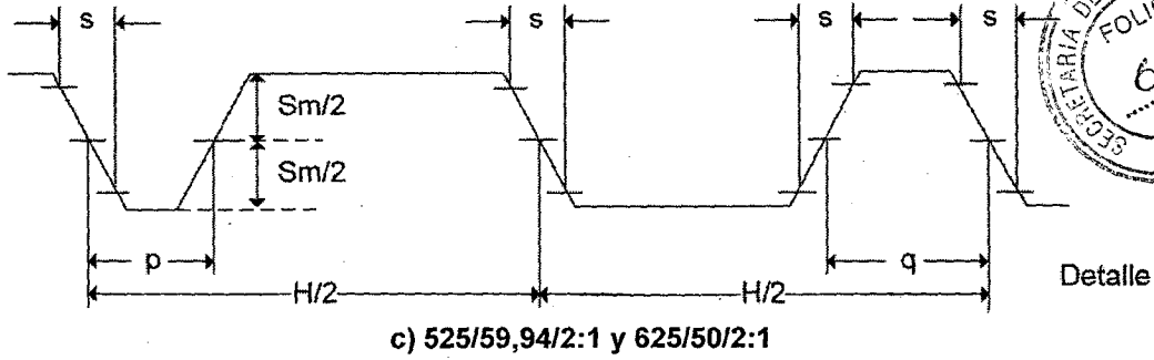
Figura 10. Señales de sincronismo de campo para 525/59,94/2:1 y 625/50/2:1
