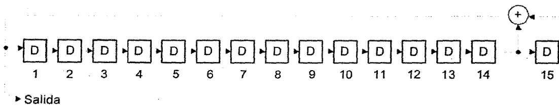
Figura 10. Generación del polinomio PRBS y circuito
