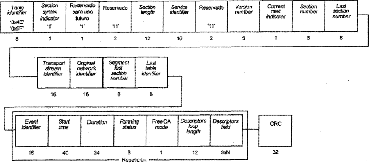
Figura 7. Estructura de datos de la EIT
