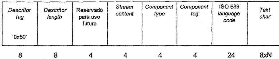
Figura 32. Estructura de datos del descriptor de componentes
