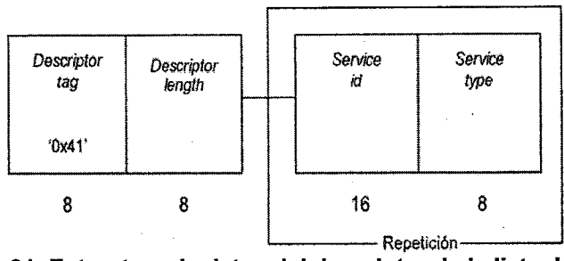
Figura 21. Estructura de datos del descriptor de la lista de servicios
