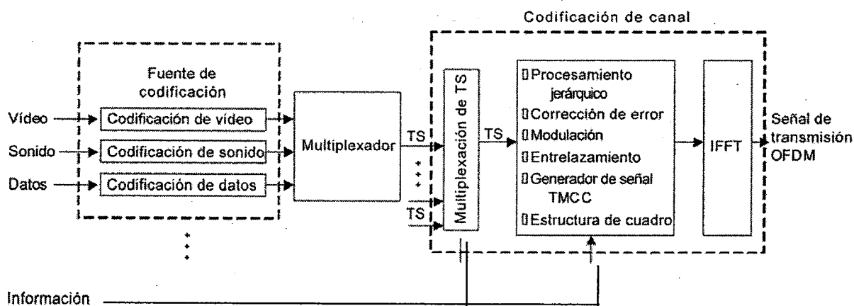
Diagrama en bloques del sistema de transmisión
