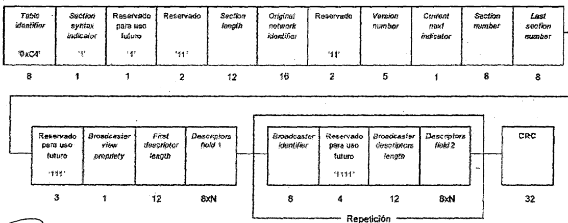
Figura 16. Estructura de datos de la BIT
