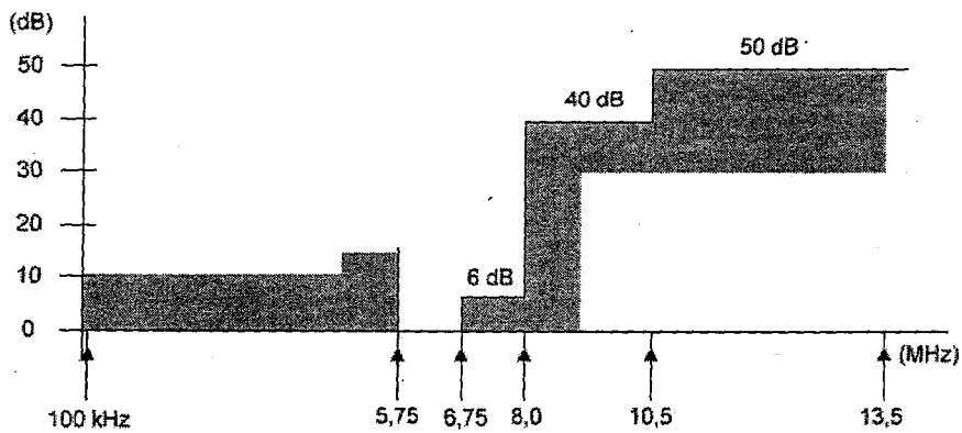
Figura 4. Características de atenuación vs. frecuencia para las señales de complemento de color en los filtros del sistema 525/59,94/1:1 y 625/50/1:1 (atenuación relativa a la de 100 kHz)
