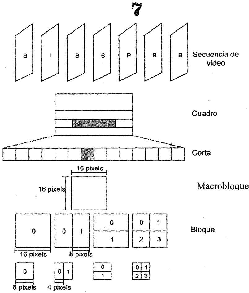
Figura 15. Fraccionamiento de la secuencia de video en macrobloques
