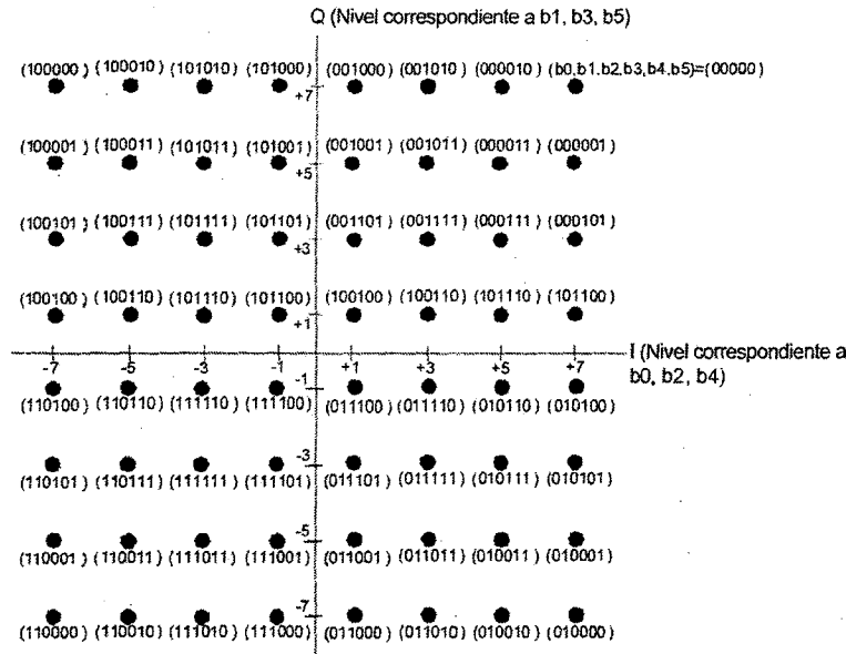
Figura 21. Constelación 64QAM
