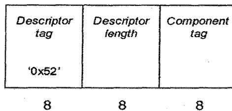
Figura 33. Estructura de datos del descriptor de identificación
