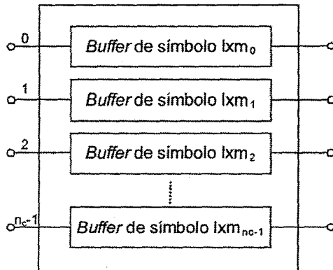
Figura 25. Configuración de la sección de time interleaving intra data
