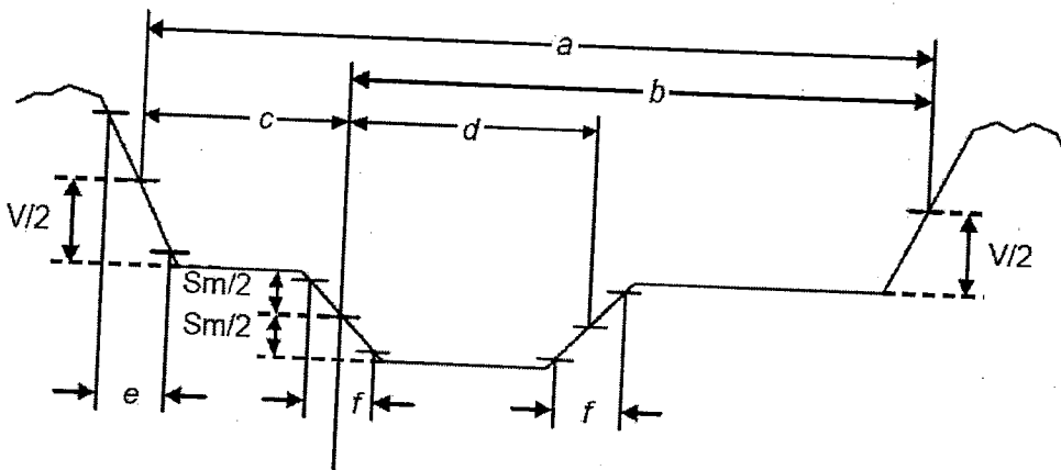
Figura 7. Señal de sincronismo de línea para 525/59,94/2:1, 525/59,94/1:1, 625/50/2:1 y 625/50/1:1
