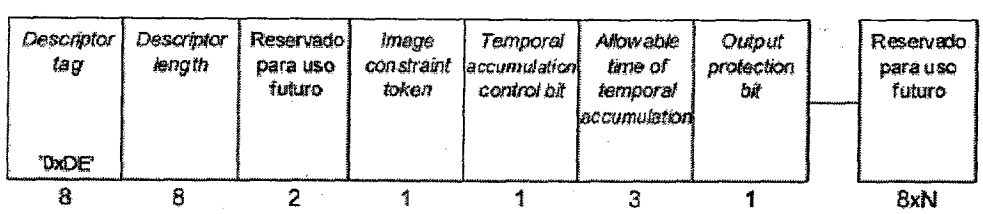
Figura 68. Estructura de datos del descriptor de disponibilidad de contenido
