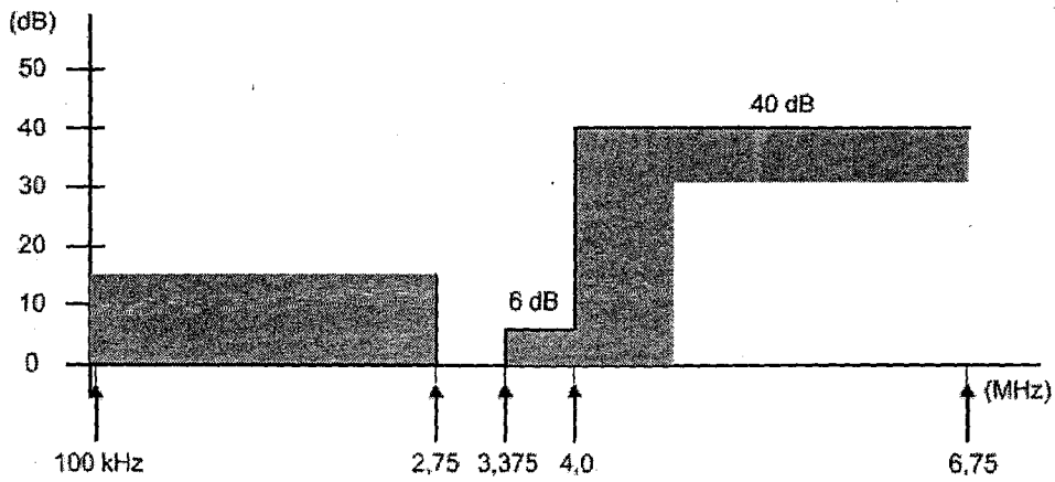
Figura 2. Características de atenuación vs. frecuencia para las señales de complemento de color en los filtros del sistema 525/59,94/2:1 y 625/50/2:1 (atenuación relativa a la de 100 kHz)
