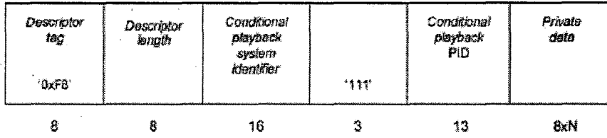
Figura 70. Estructura de datos del descriptor de reexhibición condicional
