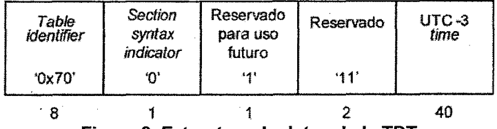
Figura 8. Estructura de datos de la TDT
