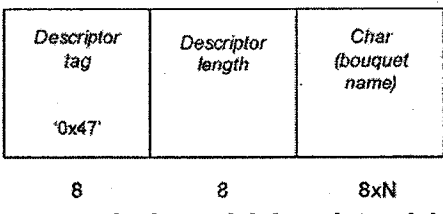
Figura 23. Estructura de datos del descriptor del nombre del ramo
