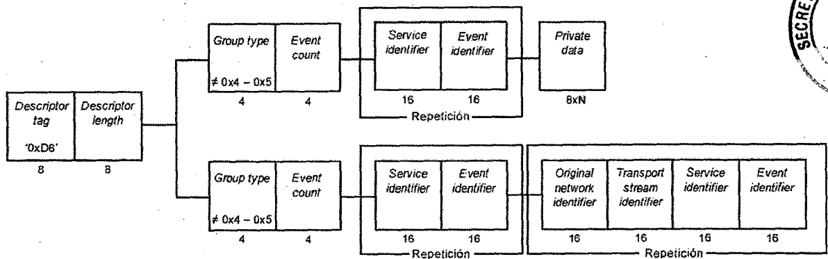
Figura 57. Estructura de datos del descriptor de grupos de eventos
