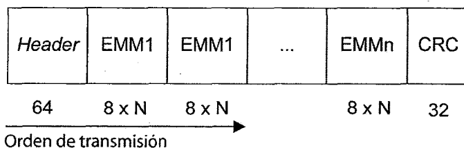
Figura 30. Estructura y procedimiento de transmisión de la EMM
