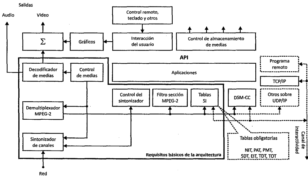
Figura 4- Arquitectura básica del receptor
