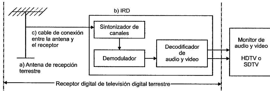
Figura 1. Configuración básica del receptor
