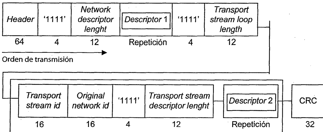
Figura 28. Tabla de información de red
