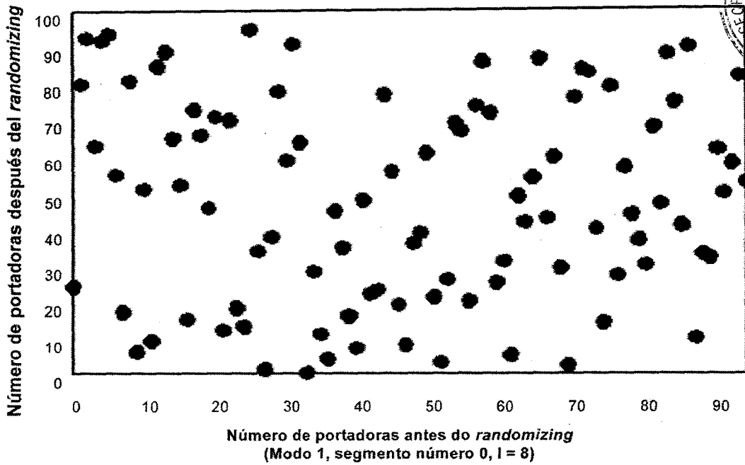
Figura 30. Ejemplo de arreglo de las portadoras antes y después del randomizing de las portadoras
