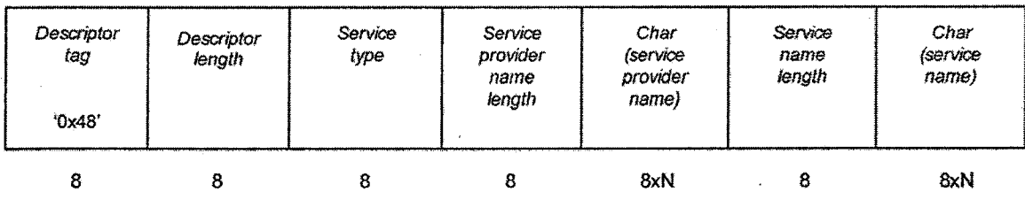
Figura 24. Estructura de datos del descriptor del servicio
