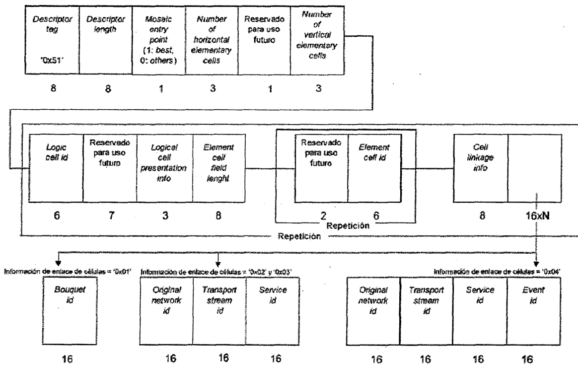
Figura 32. Estructura de datos del descriptor de mosaico
