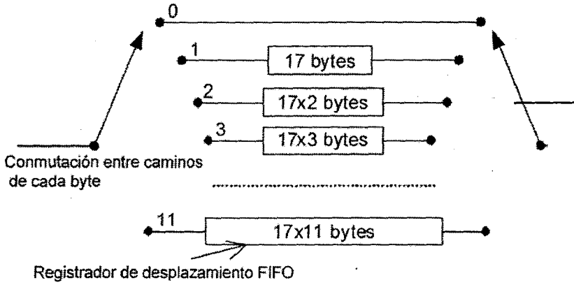
Figura 11. Circuito de byte interleaving
