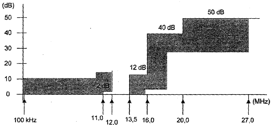
Figura 3. Características de atenuación vs. frecuencia para la señal de luminancia en los filtros del sistema 525/59,94/1:1 y 625/50/1:1 (atenuación relativa a la de 100 kHz)
