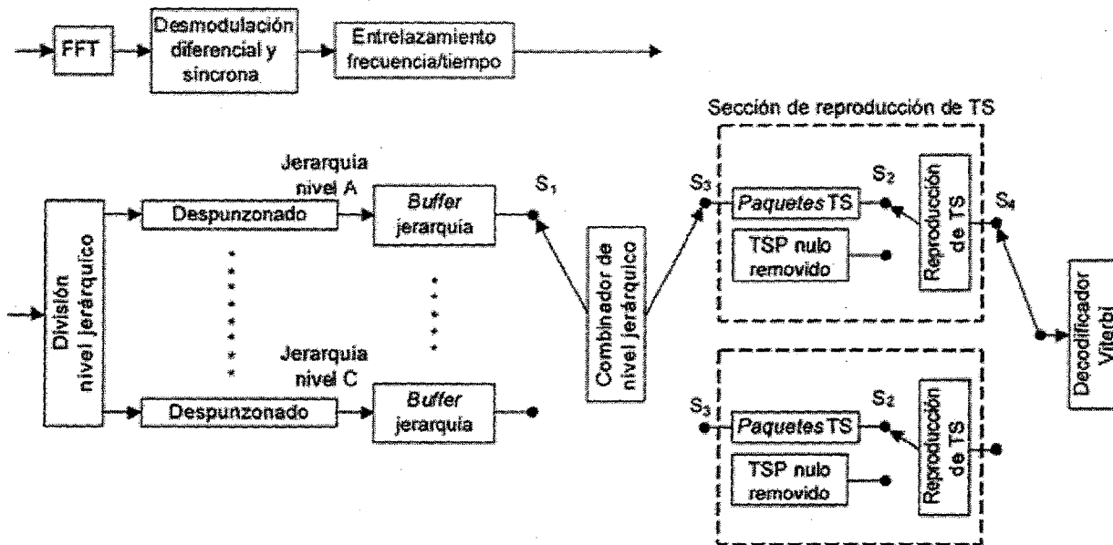
Figura 6. Modelo de receptor para referencia de cuadro múltiple
