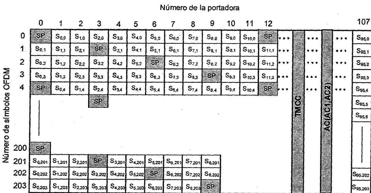
Figura 33 Configuración del segmento OFDM para modulación síncrona (QPSK, 16QAM, 64QAM) en el modo 1
