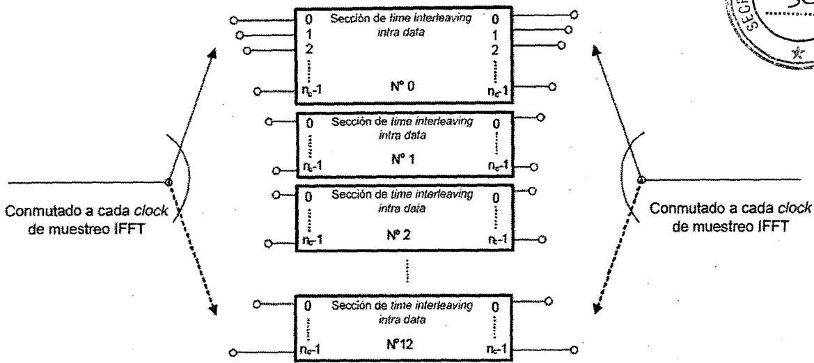
Figura 24. Configuración de la sección de entrelazamiento en tiempo
