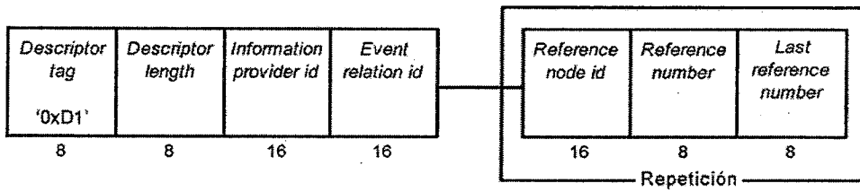
Figura 50. Estructura de datos del descriptor de referencia
