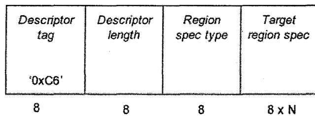
Figura 46. Estructura de datos del descriptor de región meta
