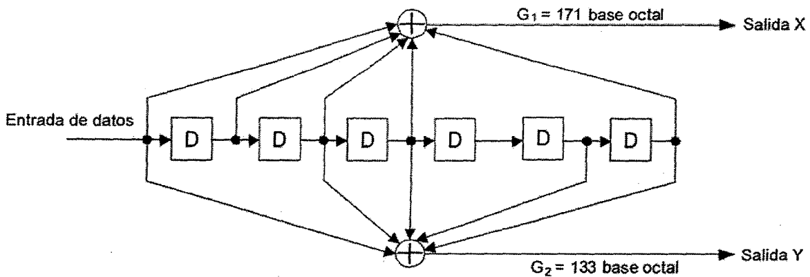
Figura 12. Circuito de codificación del código convolucional con profundidad k de 7 y tasa de codificación de 1/2
