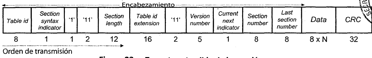
Figura 23. Formato extendido de la sección
