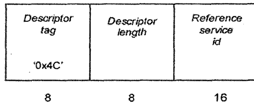
Figura 28. Estructura de datos del descriptor de horario de cambio de servicio (Time shifted)
