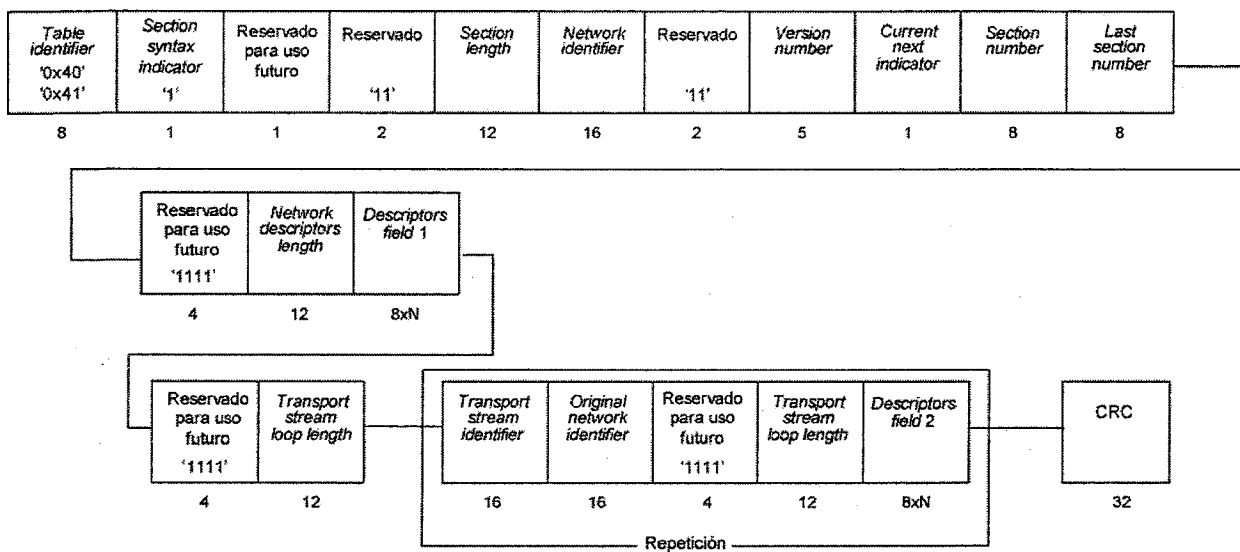
Figura 4. Estructura de datos de la NIT
