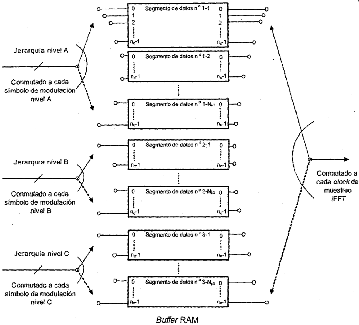
Figura 23. Configuración del combinador de capas
