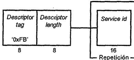
Figura 55. Estructura de datos del descriptor de recepción parcial
