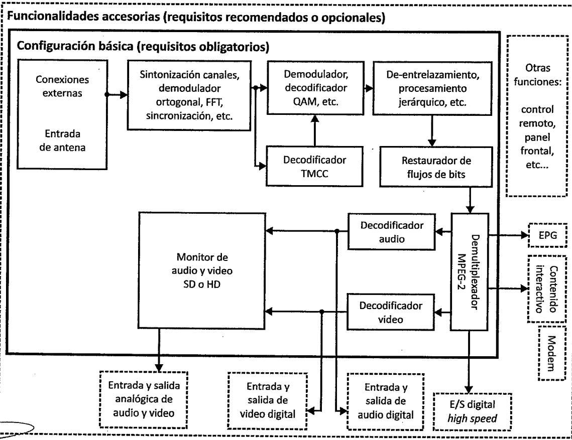
Figura 2-Configuración básica del IRD tipo convertidor digital (STB)
