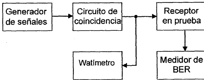
Figura C.1 – Método de medición del nivel de entrada
