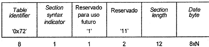
Figura 11. Estructura de datos de la ST
