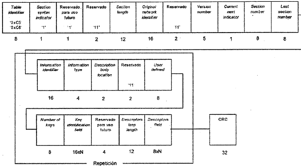
Figura 17. Estructura de datos de la NBIT
