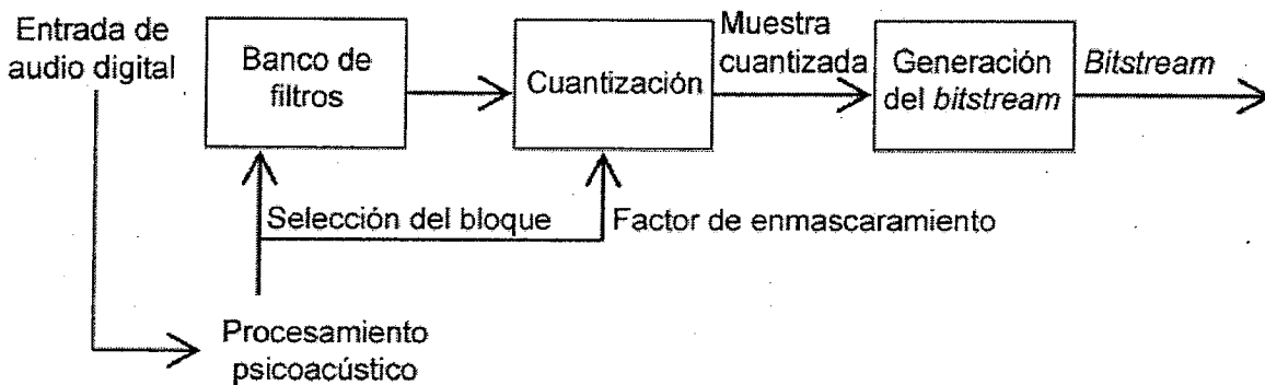
Figura 17. Procedimientos de transmisión y codificación de audio
