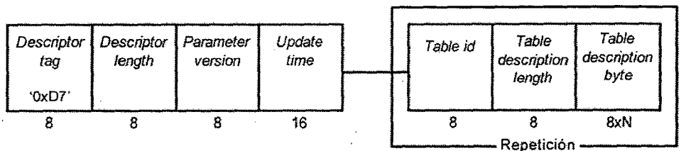
Figura 58. Estructura de datos del descriptor de parámetro de SI
