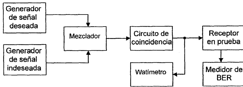
Figura C.2 – Método de medición de la selectividad
