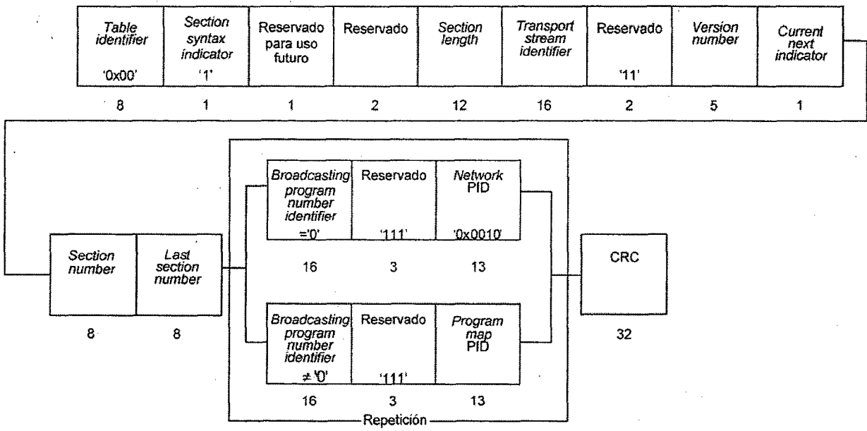
Figura 1. Estructura de datos de la PAT
