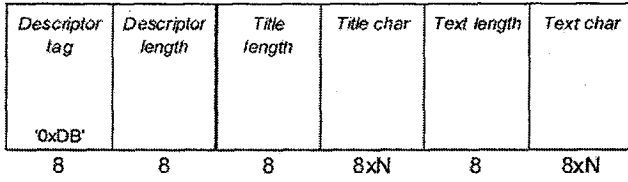
Figura 62. Estructura de datos del descriptor de la información incorporada
