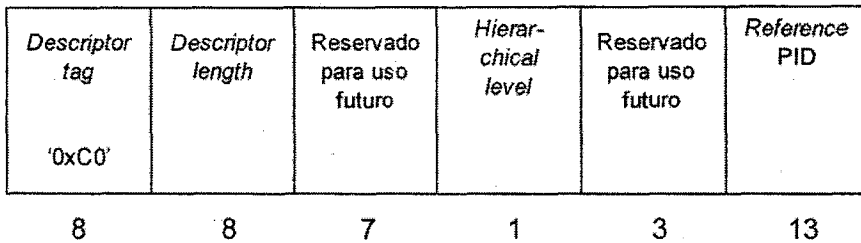
Figura 40. Estructura de datos del descriptor de transmisión jerárquica
