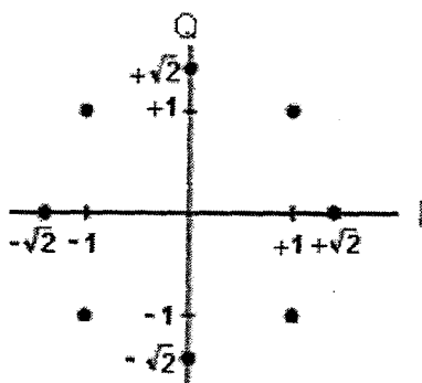
Figura 15. Constelación DQPSK - Desplazamiento \pi/4
