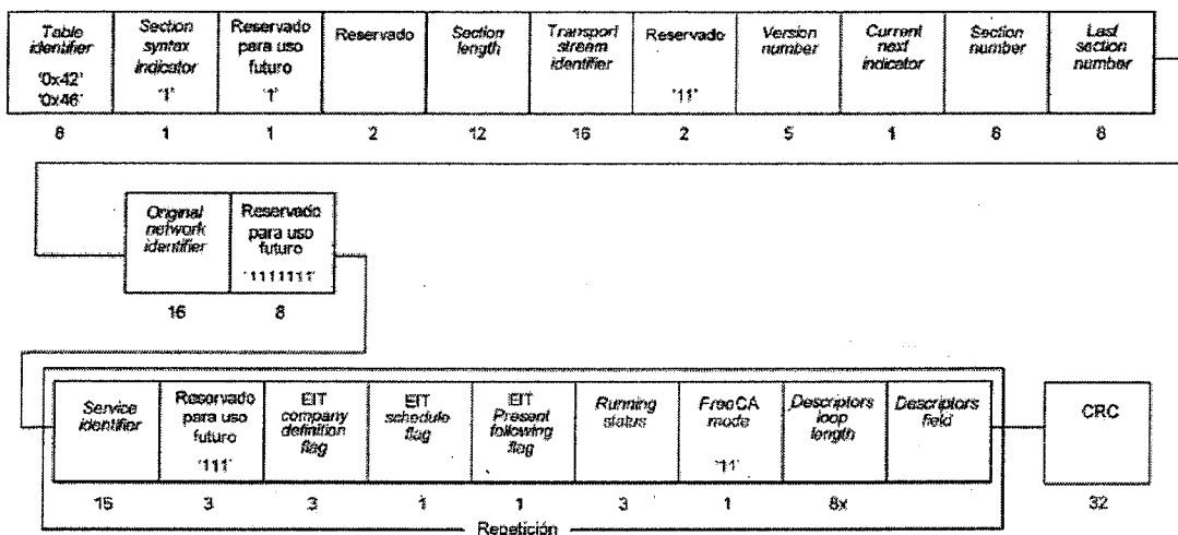
Figura 5. Estructura de datos de la SDT
