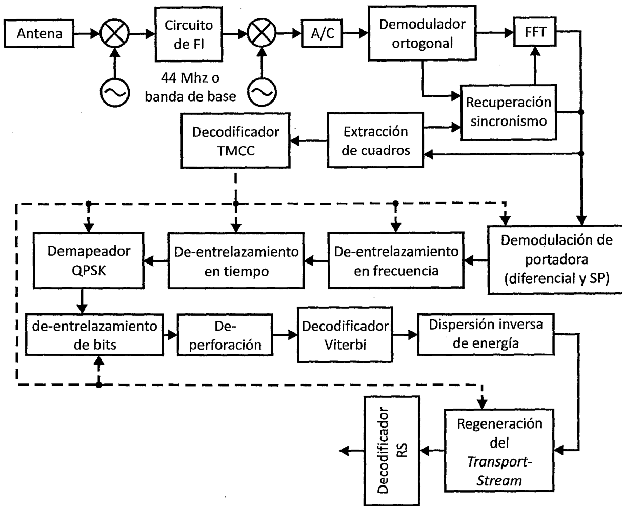
Figura 6-Procesamiento de señal en el front-end para one-seg
