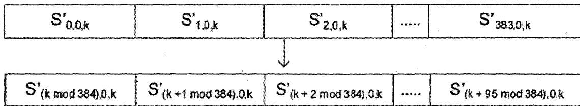
c) Rotación de portadora en el modo 3
