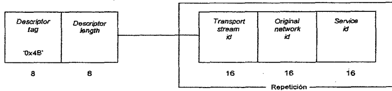
Figura 27. Estructura de datos del descriptor de referencia NVOD
