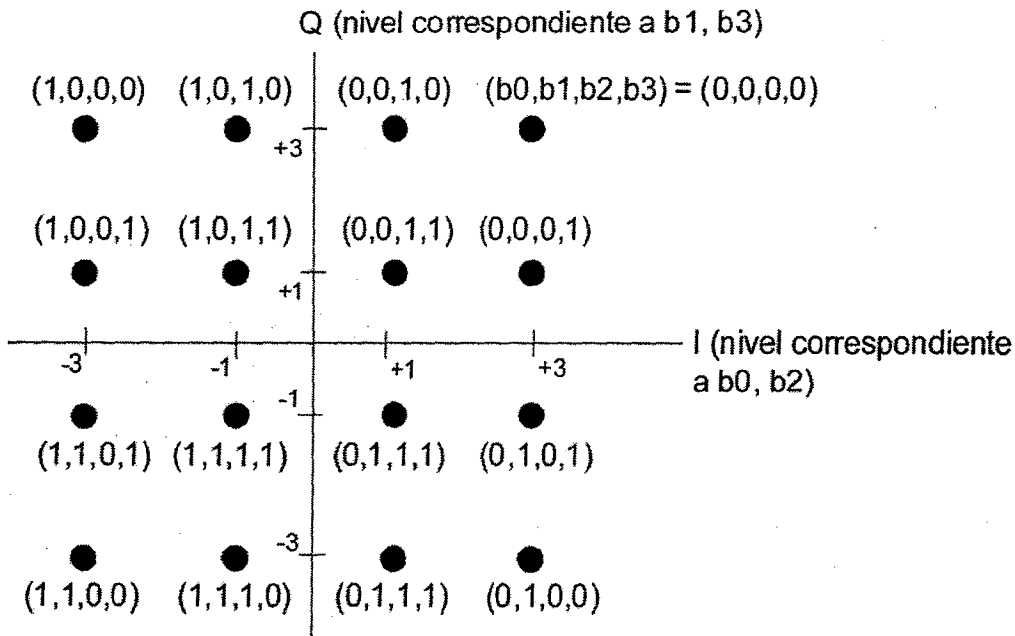
Figura 19. Constelación 16QAM
