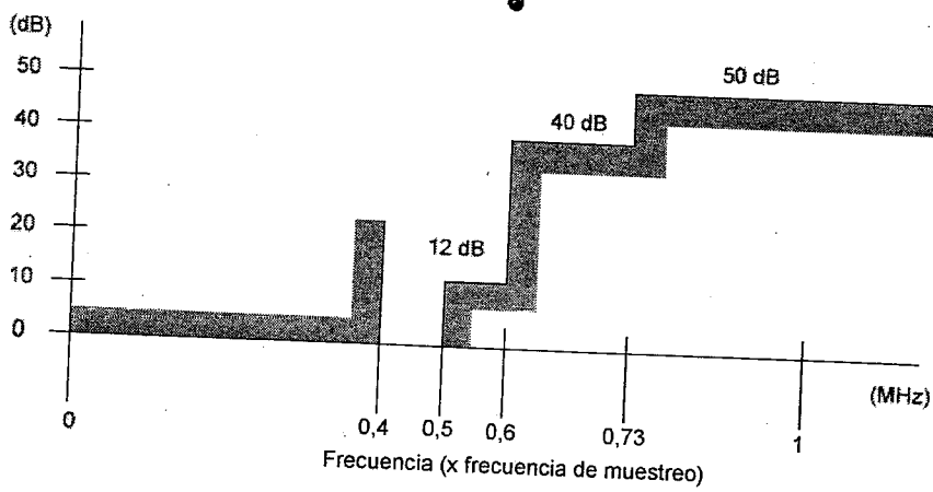
Figura 5. Características de atenuación vs. frecuencia para la señal de luminancia en los filtros de los sistemas 750/59,94/50/1:1 y 1125/59,94/50/2:1 (atenuación relativa a la de 100 kHz)
