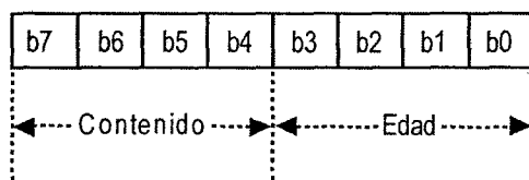
Figura 80. Distribución de los bits del campo rating
