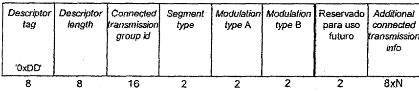
Figura 64. Estructura de datos del descriptor de transmisiones conectadas de audio
