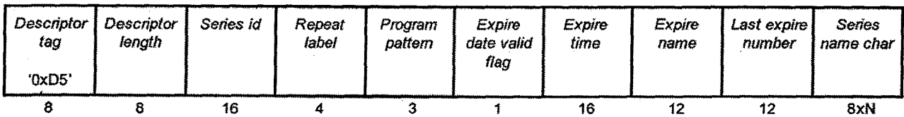
Figura 56. Estructura de datos del descriptor de series
