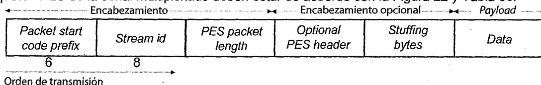
Figura 22. Estructura del paquete PES y sus secciones
