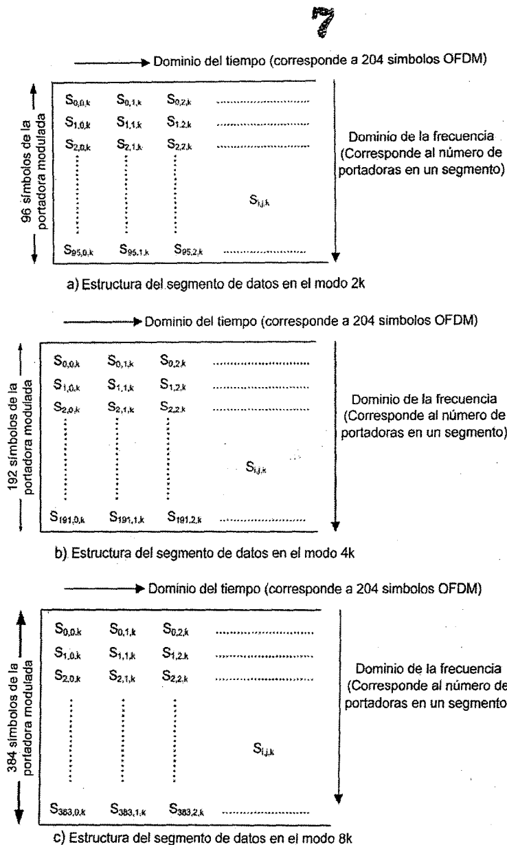
Figura 22. Configuración del segmento de datos
