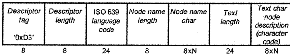
Figura 52. Estructura de datos del descriptor de información de short node
