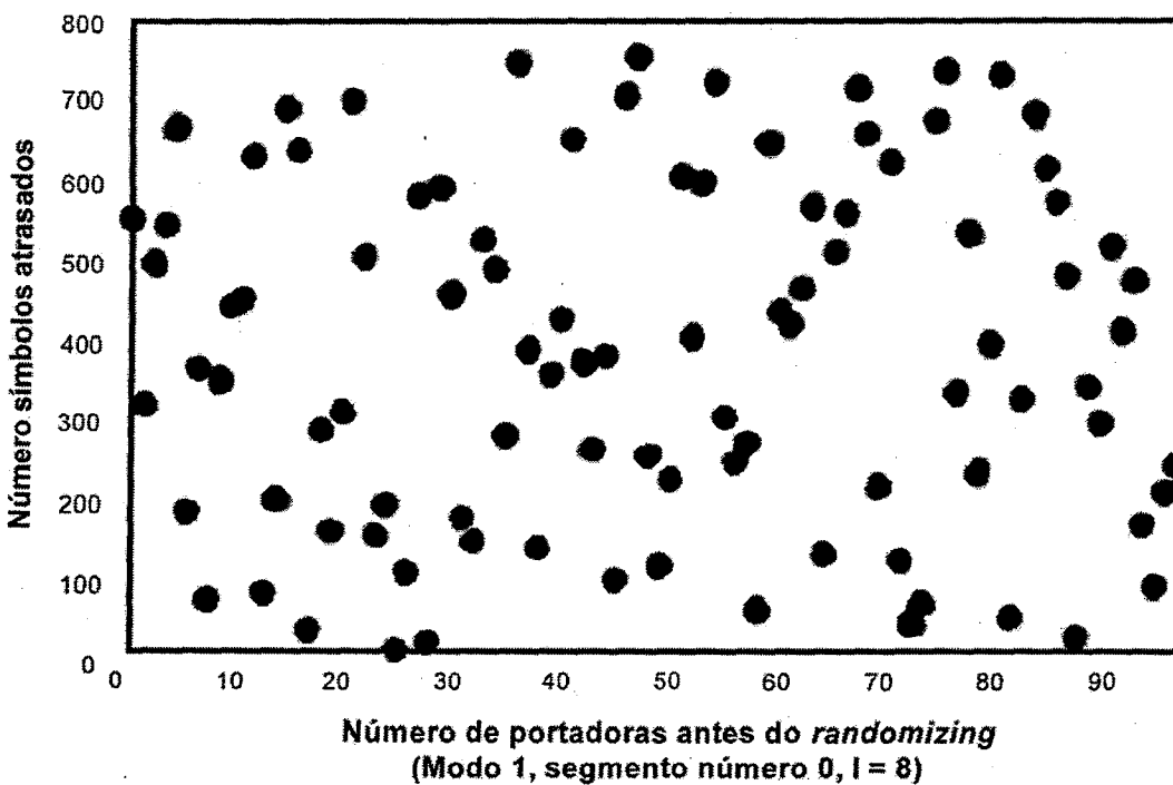
Figura 31. Ejemplo de arreglo de las portadoras después del entrelazamiento en tiempo y del randomizing de las portadoras
