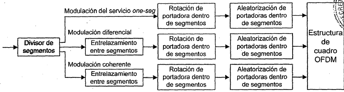
Figura 27. Configuración de la sección de entrelazamiento en frecuencia
