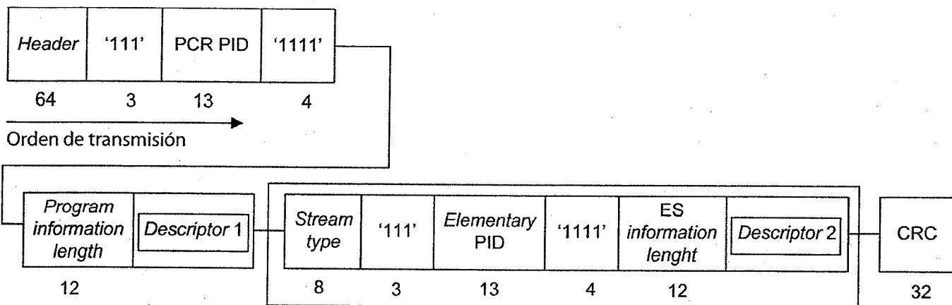
Figura 26. Tabla de mapeo de programa
