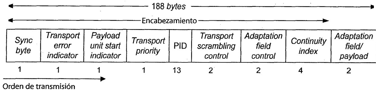
Figura 24. Estructura del paquete TS y sus secciones
