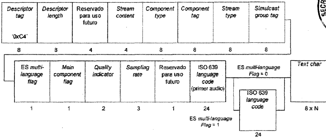
Figura 44. Estructura de datos del descriptor de componentes de audio
