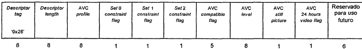
Estructura de datos del descriptor de video AVC
