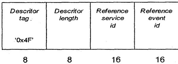
Figura 31. Estructura de datos del descriptor de horario de cambio de eventos
