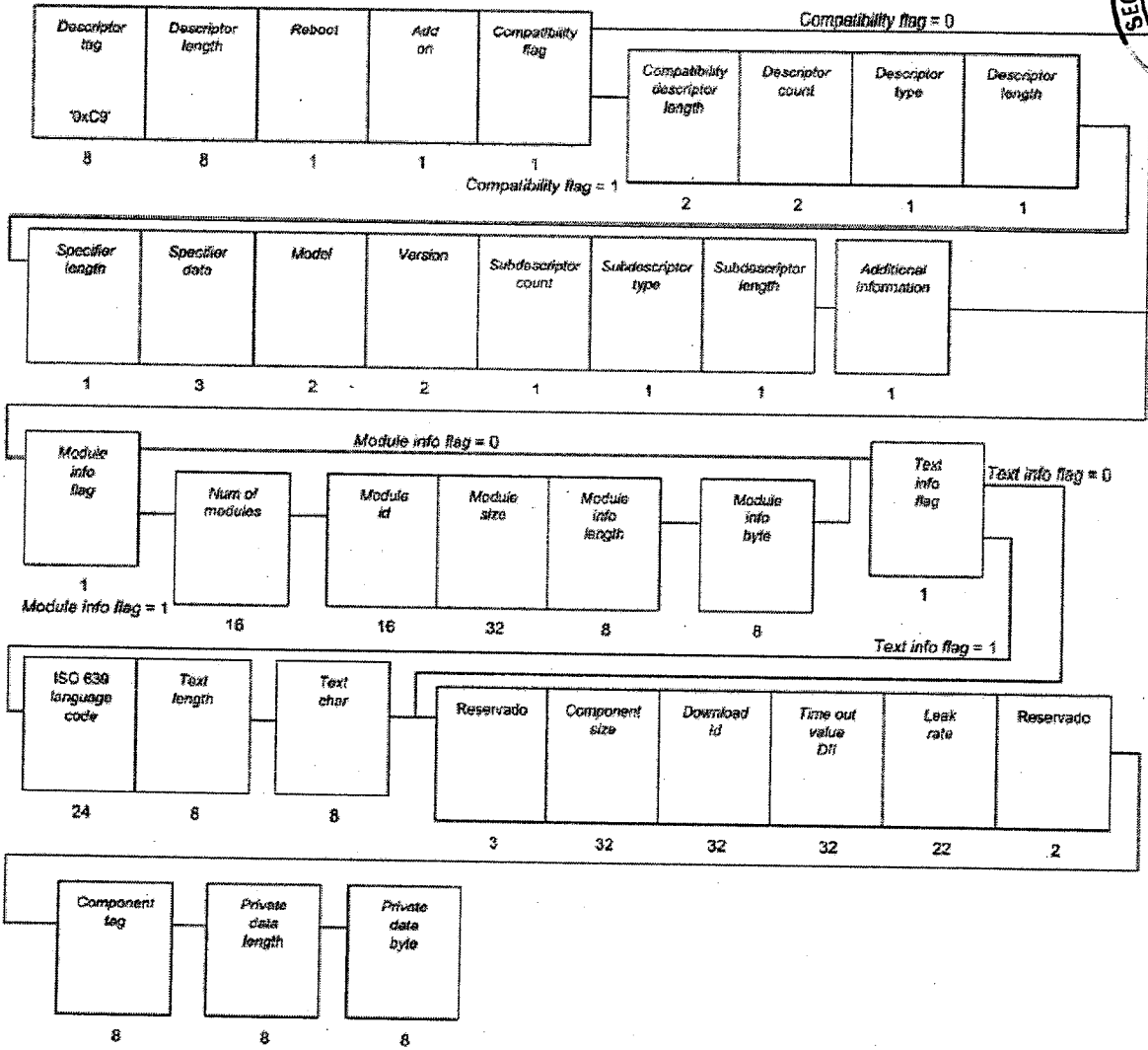
Figura 76. Estructura del descriptor de contenido de actualización de receptores
