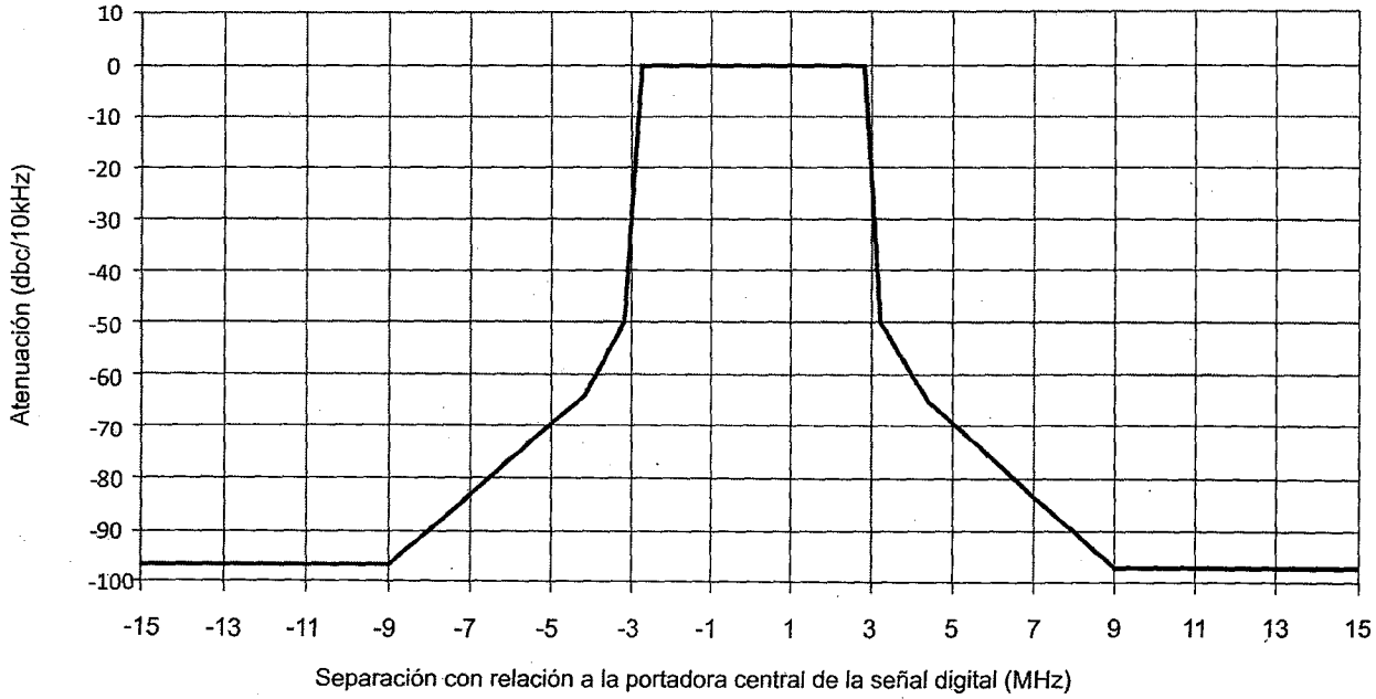
Figura 38. Máscara del espectro de transmisión para radiodifusión de televisión digital terrestre
