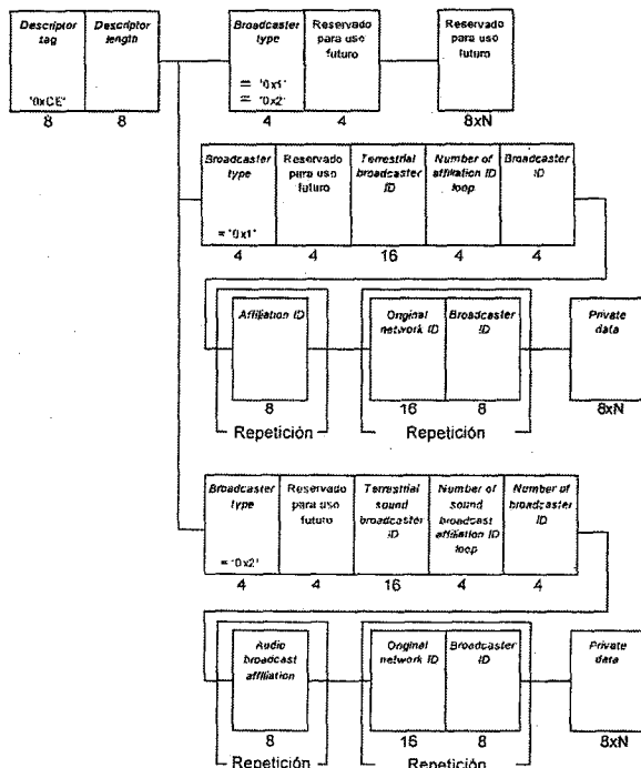
Figura 66. Estructura de datos del descriptor extendido de radiodifusión
