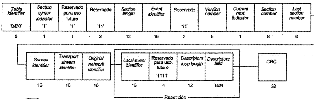
Figura 13. Estructura de datos de la LIT
