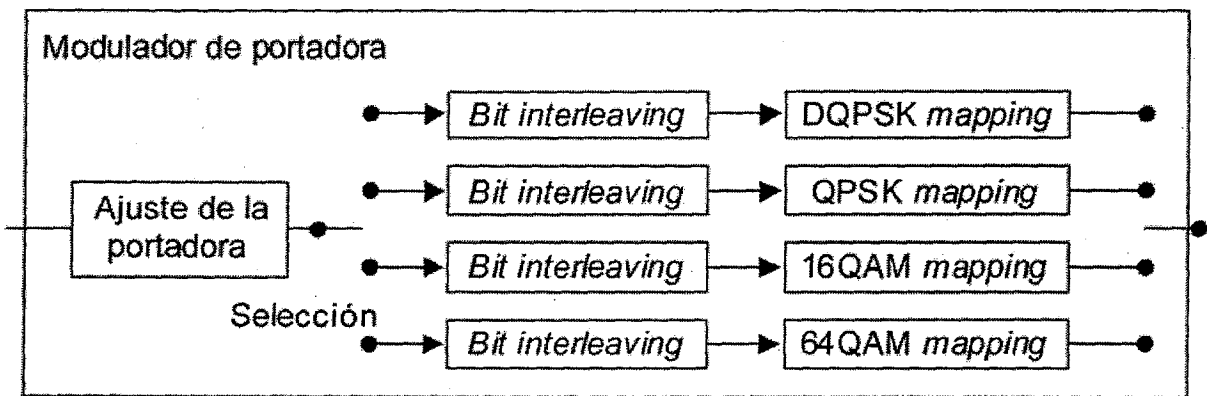
Figura 13. Configuración de la modulación de la portadora
