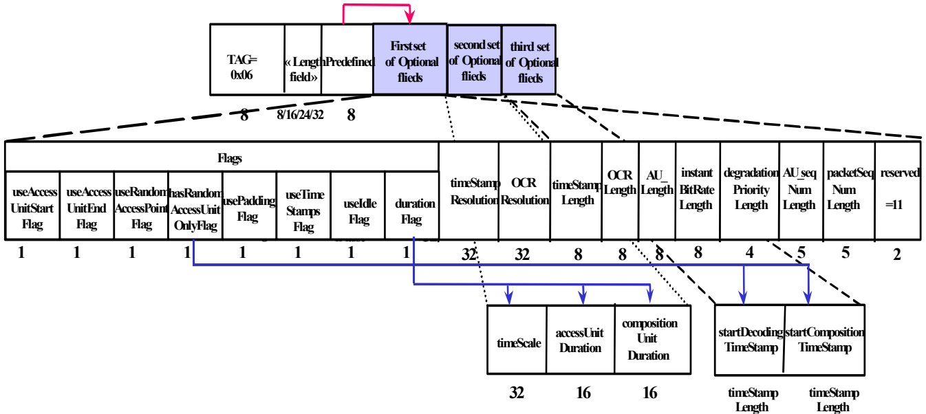
SLConfigDescriptor
